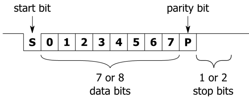
Figure 17. Modbus message frame
